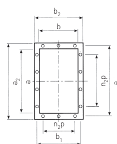
Flangia premante Discharge flange
