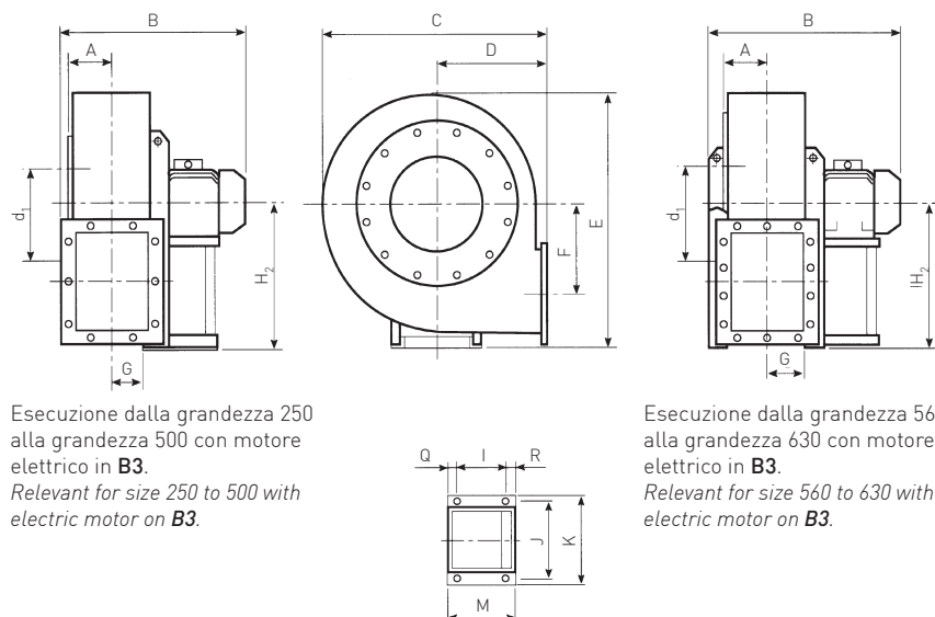
Forature sedia di sostegno motore elettrico Drill holes on motor support frame
